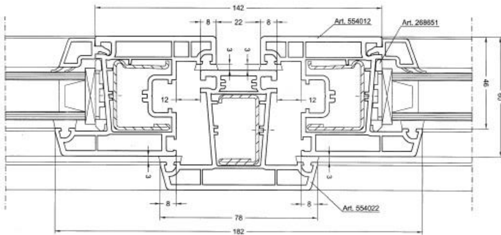
Sezione nodo Euro 60 .1
